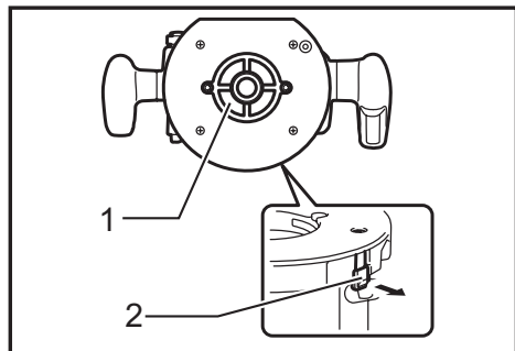
► 1. Guide de gabarit 2. Plaque de verrouillage
