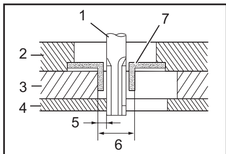
► 1. Punta de atornillar 2. Base 3. Plantilla 4. Pieza de trabajo 5. Distancia (X) 6. Diámetro exterior de la guía de plantilla 7. Guía de plantilla
