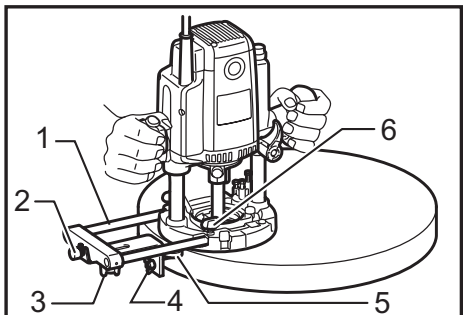
► 1. Porte-guide 2. Vis de réglage 3. Vis de serrage (B) 4. Vis de serrage (C) 5. Guide d'affleurage 6. Vis de serrage (A)
