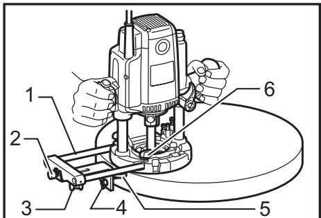
► 1. Portagúa 2. Tornillo de ajuste 3. Tornillo de sujeción 4. Tornillo de sujeción (C) 5. Guía de recorte 6. Tornillo de sujeción (A)
