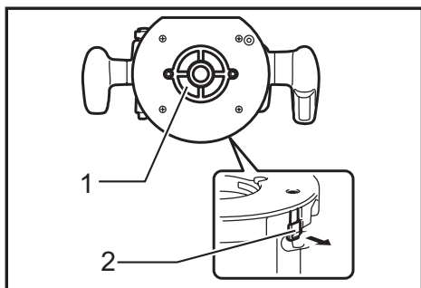
► 1. Template guide 2. Lock plate
